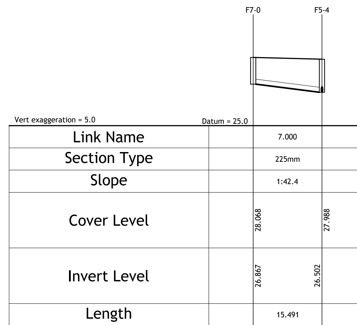
PIPERUN F7
