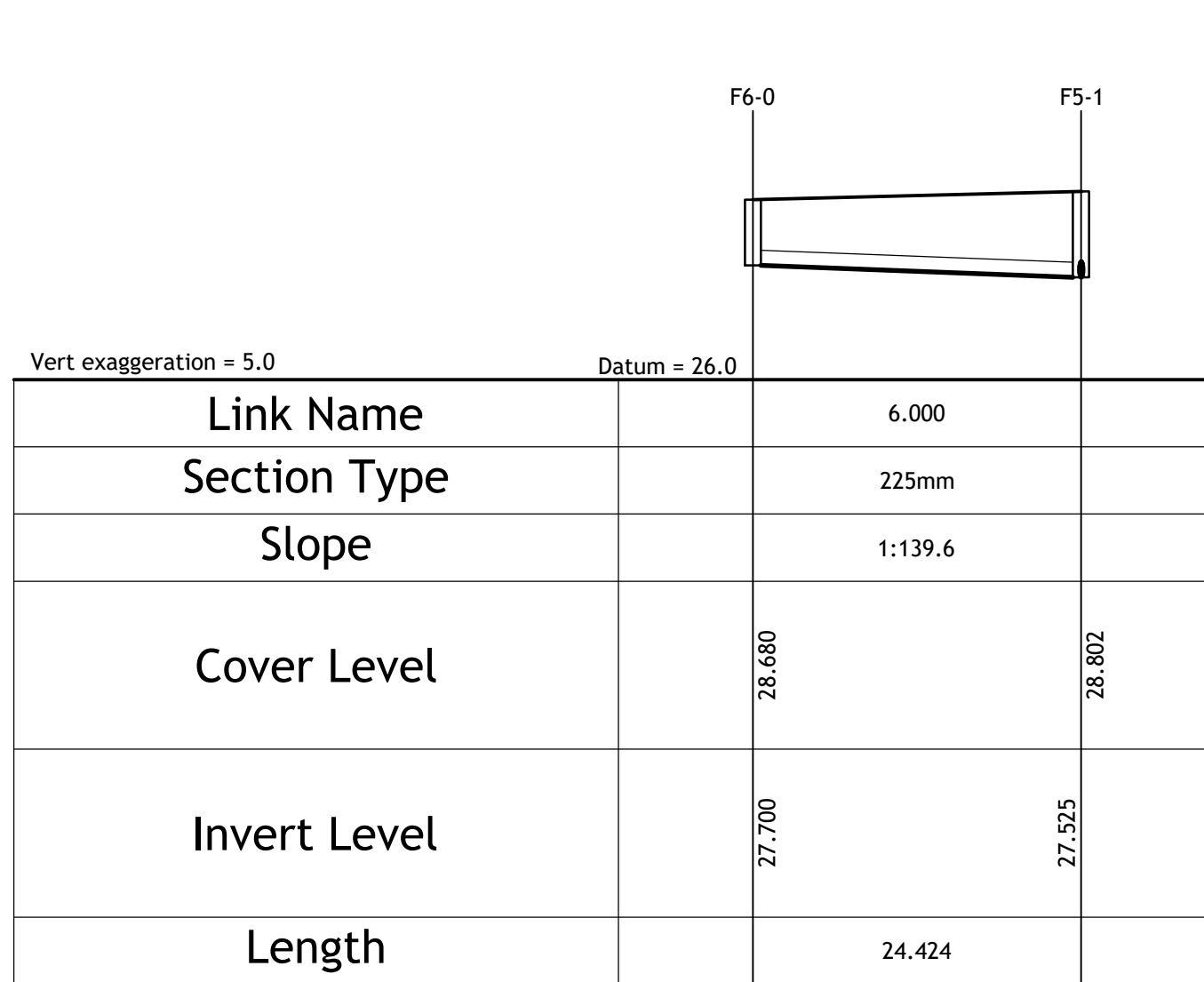
PIPERUN F6
